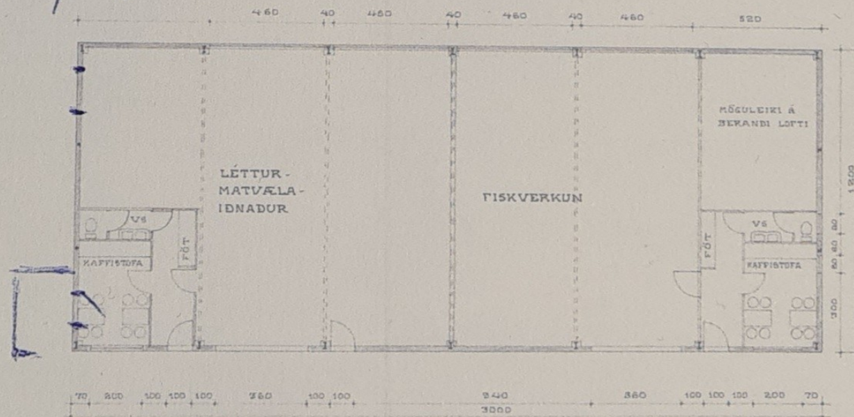
GRUNNMYND M. 1:100
