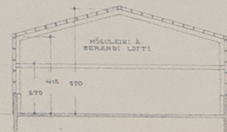
SNID M. 1:100
