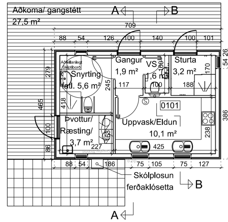
GRUNNMYND, 1:100
